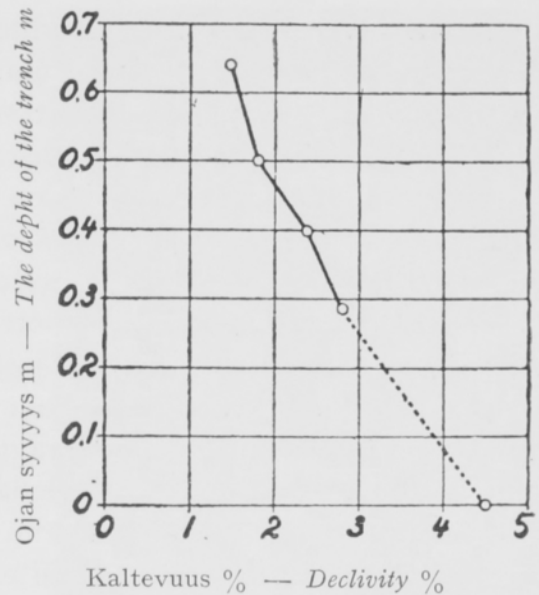
Kuva 10. Ojan syvyyden riippuvaisuus maanpinnan kalvetuudesta Suomessa.
