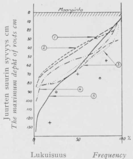
Kuva 4. Lukuisuuskäyriä eri viljelyskasvien juurten suurimmasta syvyydestä Suomessa SALOSEN mittausten mukaan. 1 = nurmikasvit paitsi apila, 2 = peruna, 3 = kevätvilja, 4 = ruis, 5 = apila. Ristit esittävät syysvehnän ja pienet ympyrät sokerijuurikkaan yksityisiä havaintoja.
