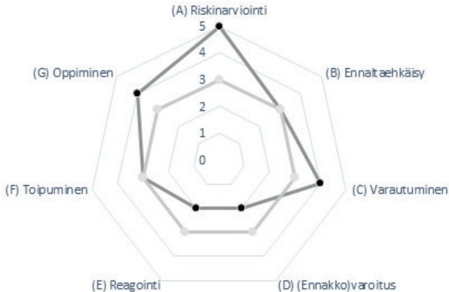
Kuvio 3. CIRI-tulosten havainnollistaminen (sovellus Rød ym. 2020 mukaan). Vaaleanharmaa kuvaa minimitasoa, tumma mittaus tuloksia.
