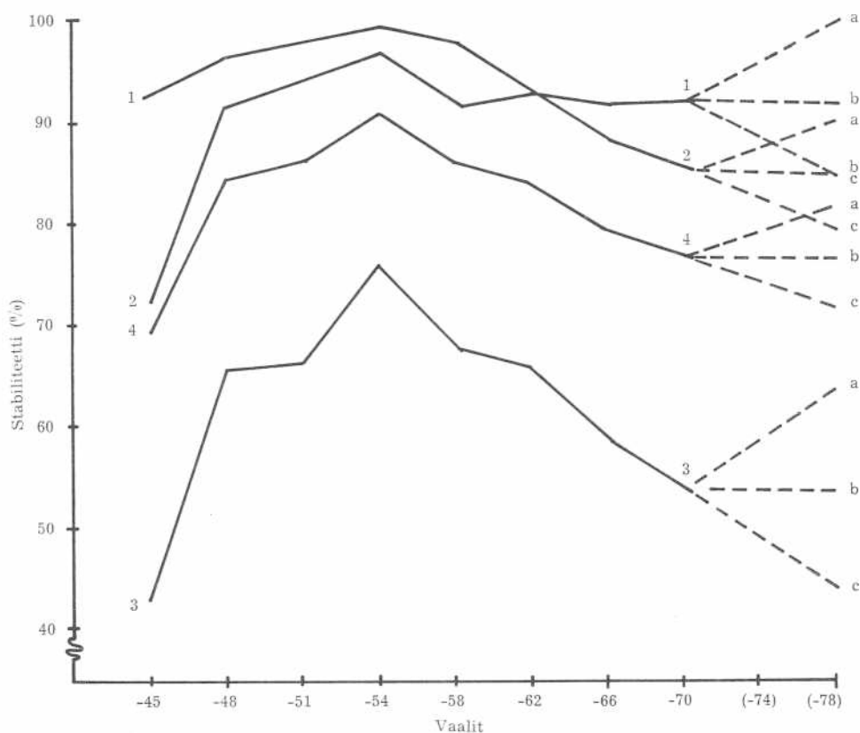
Kuvio 2. Vasemmisto — oikeisto -stabiiliteetin (1), puolueiden voimasuhteiden stabiiliteetin (2), henkilöstabiiliteetin (3) sekä kokonaisstabiiliteetin (4) kehitys vuosina 1945—1970 ynnä tulevan kehityksen ennakointi.
