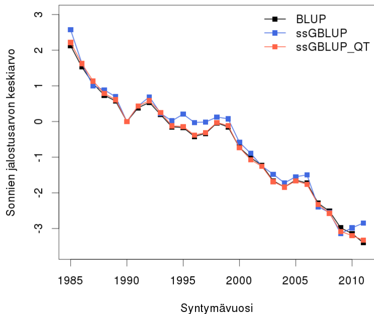
Kuva 3. Kolmannen lypsykauden uusimattomuusprosentin jalostusarvojen korrelaatiot syntymävuosittain lehmillä (F) ja sonneilla (M) sekä perinteisen eläinmallin ja genomisen eläinmallin välillä (BLUP v. ssGBLUP) että perinteisen eläinmallin ja QT-muunnosta käyttävän genomisen eläinmallin välillä (BLUP v. ssGBLUP_QT).
