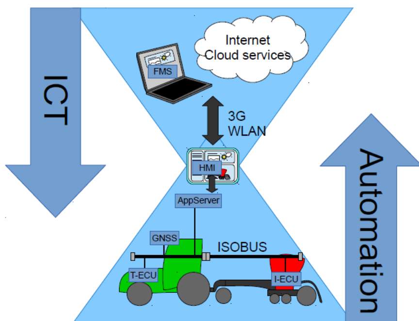
Kuva 1. Teollisen Internetin teknologiat mahdollistavat kokonaisvaltaisen järjestelmäintegraation maataloudessa yhdistämällä koneautomaation ja pilviteknologiat ratkaisut geneerisellä tavalla. (Pierros Juha Backman).
