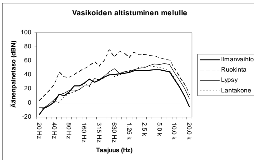
Kuva 2: Melutapahtumien spektrit 20 Hz – 20 kHz taajuuksilla N-painotettuna terssispektrinä.
