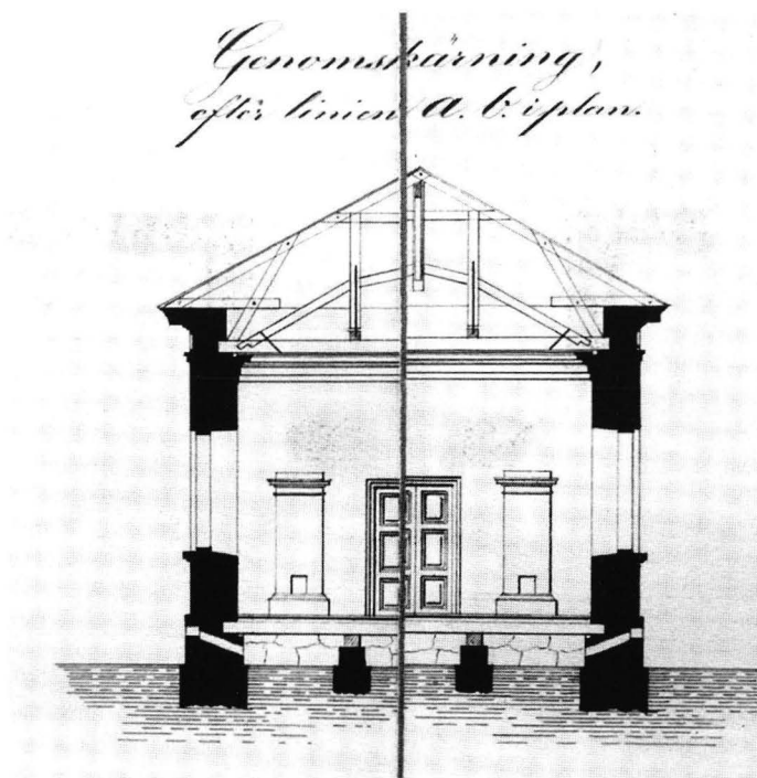
Kuva 5. Gustavsonin suunnitelma, poikkileikkaus.
