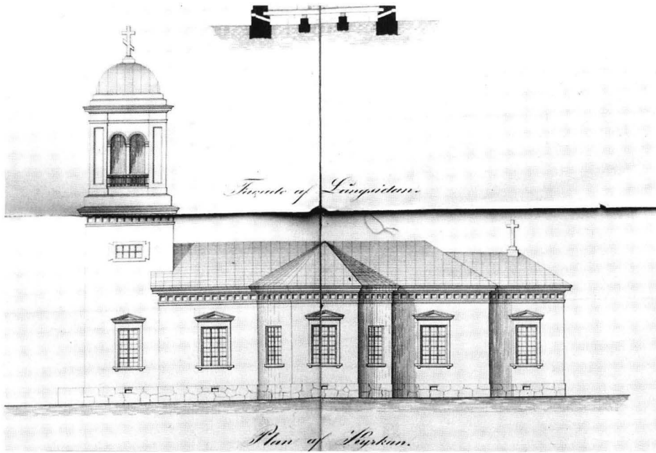
Kuva 4. Gustavsonin suunnitelma, eteläfasadi.
