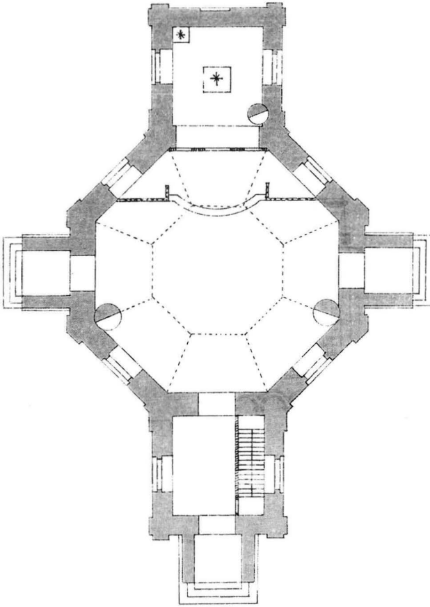
Kuva 13. Kirkon pohjakaava venäläisestä mallipiirustuskirjasta. A. M. Sadko, Rukovodstvo k ustrojstvu kamennyh i derevjannyh tserkvej (1892), numeroimaton piirros.
