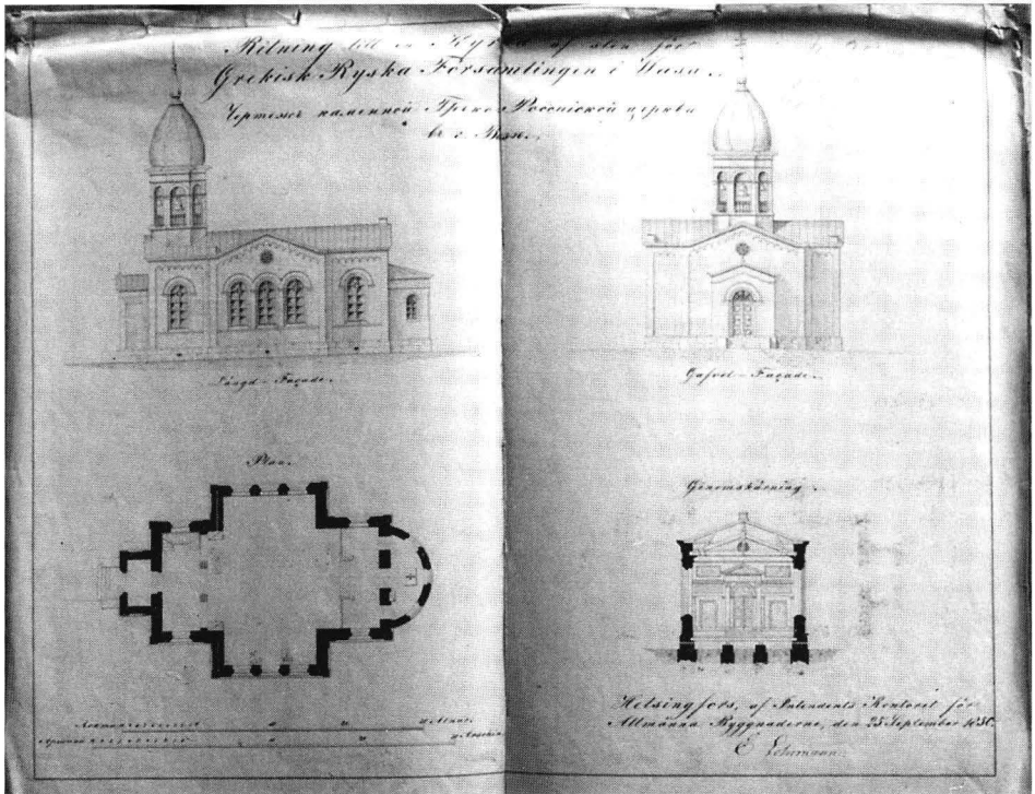
Kuva 6. E. B. Lohrmannin suunnitelma Vaasan ortodoksiseksi kirkoksi.
