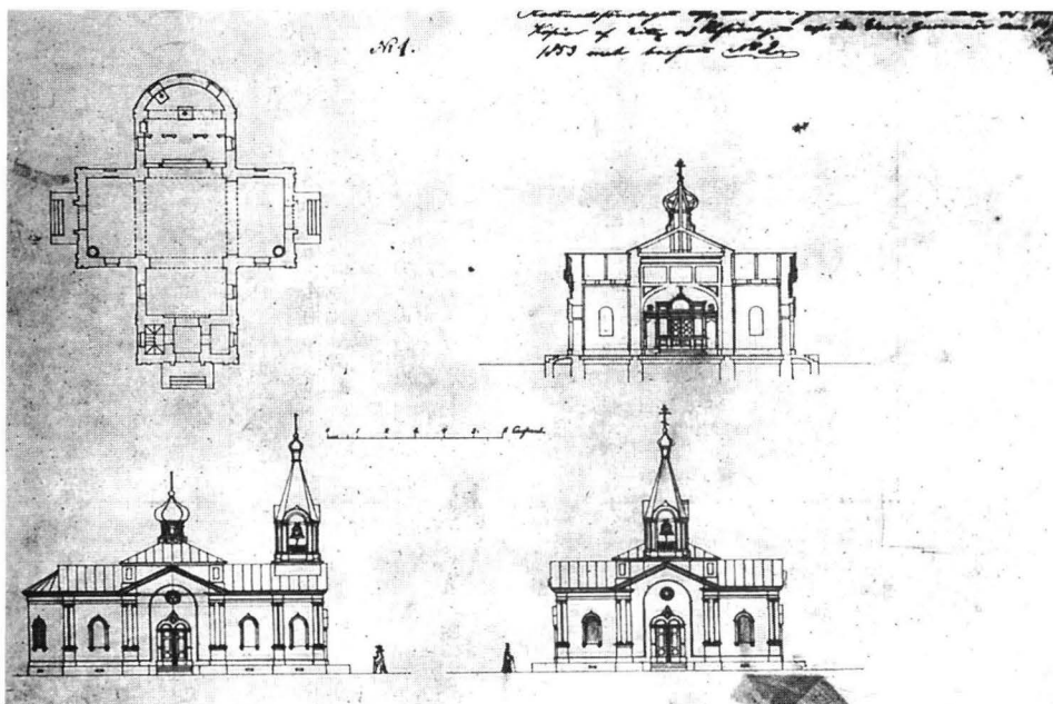
Kuva 17. Kudinovin vaihtoehtoinen suunnitelma (2), Åkerfeldtin kokoelma.
