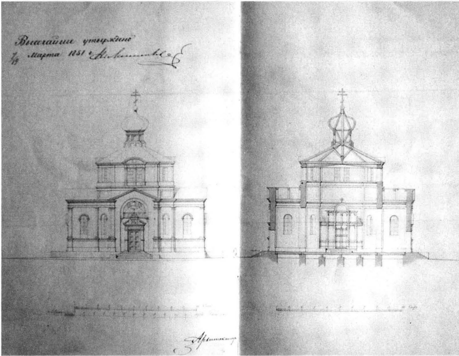
Kuva 10. A. S. Kudinovin suunnitelma Vaasan ortodoksiseksi kirkoksi. Kuvat 10–12: VSV, akti 20/1852.
