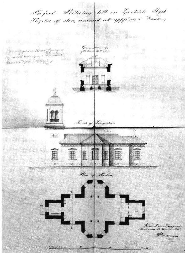
Kuva 3. Carl E. J. Gustavsonin suunnitelma Vaasan ortodoksiseksi kirkoksi. Poikkileikkaus, eteläfasadi ja pohjakaava. Kuvat 3–7: KA, KKK akti 32/1846.
