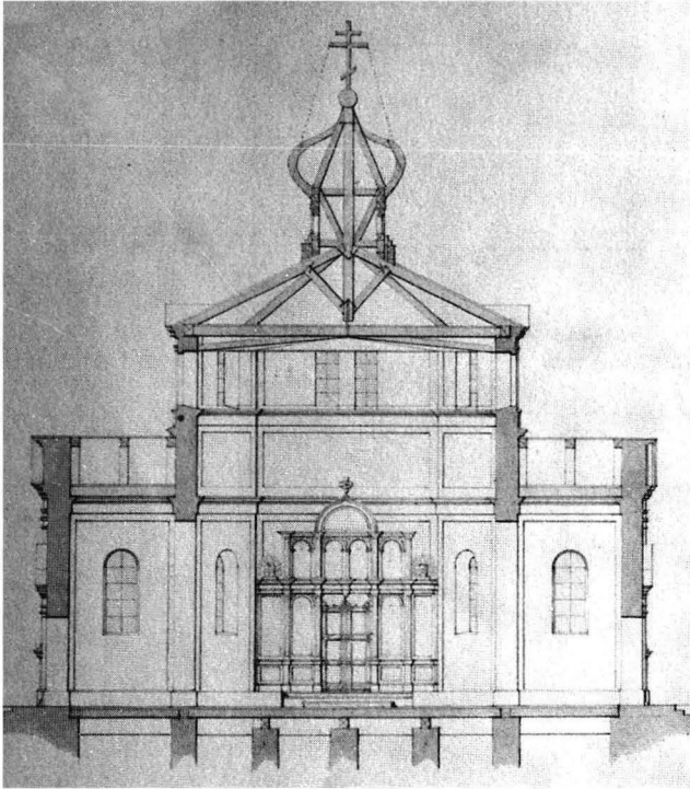
Kuva 11. Kudinovin suunnitelma, fasadi.
