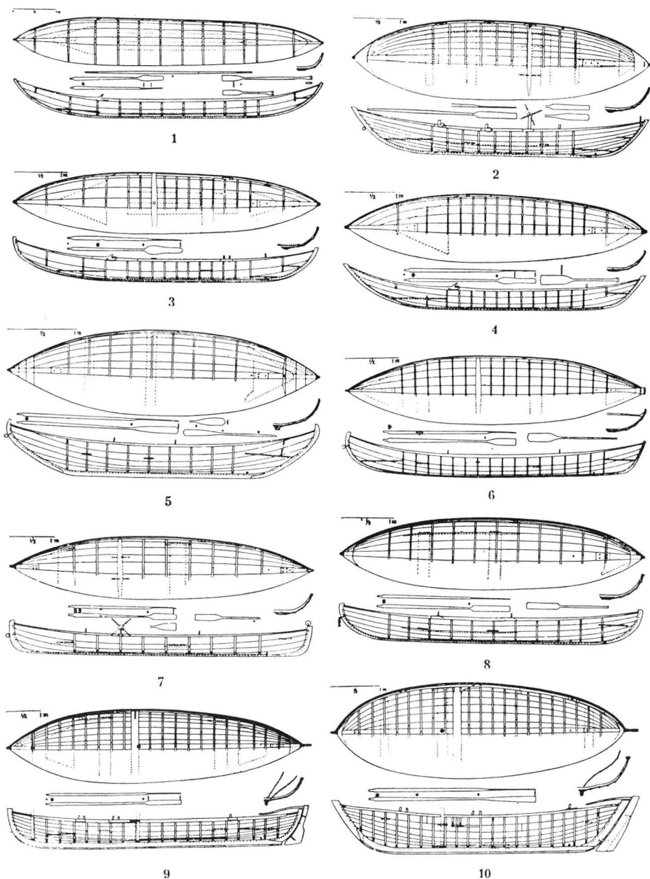
1. Peräpohjan vene. 2. Etelä-Pohjanmaan vene. 3. Kajaanin kihlakunnan vene. 4. Karjalan vene. 5. Laatokan vene. 6. Savolainen vene. 7. Hämmäläinen vene. 8. Satakuntalainen vene. 9. Pohjoinen merivene. 10. Eteläinen merivene.
