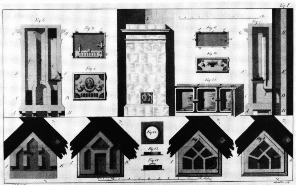
Kuva 2. Venäläinen uuni. C. L. Engelin kuvitusta teokseen Anleitung zum Bau des Russischen Stubenofens (Berlin 1821), Tafel I.
