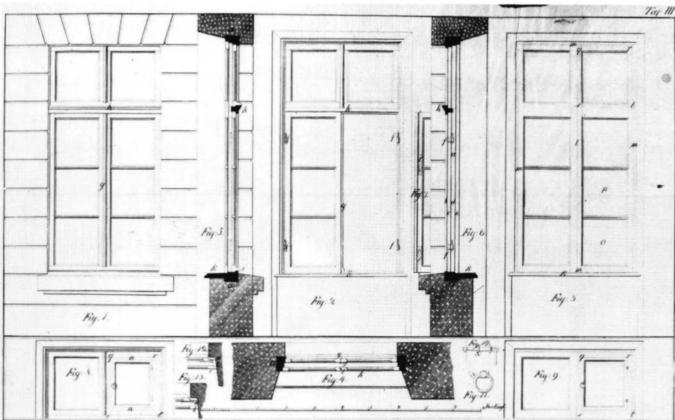
Kuva 4. Kaksinkertainen ikkuna. C. L. Engelin kuvitusta teokseen Anleitung zum Bau des Russischen Stubenofens (Berlin 1821), Tafel III.
