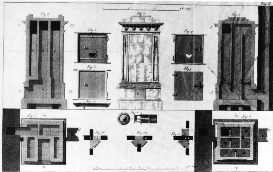
Kuva 3. Venäläinen uuni. C. L. Engelin kuvitusta teokseen Anleitung zum Bau des Russischen Stubenofens (Berlin 1821), Tafel II.
