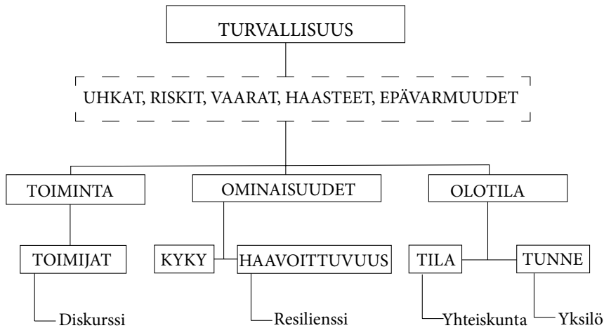
Kuva 1. Turvallisuuskäsitteen ominaispiirteet.
