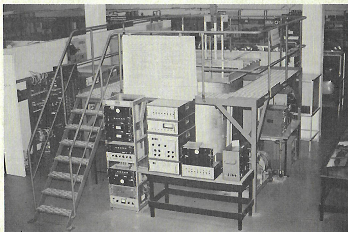
Atomivoimalan alikriittinen reaktori Sähköhallin keskellä. Se on aikanaan toiminut opetustehtävissä TKK:ssa Otaniemessä.
