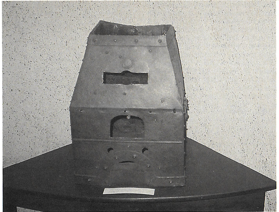
Mäntsälän Alikartanossa oleva sulatusuuni. Valok. Teuvo Nortia.
