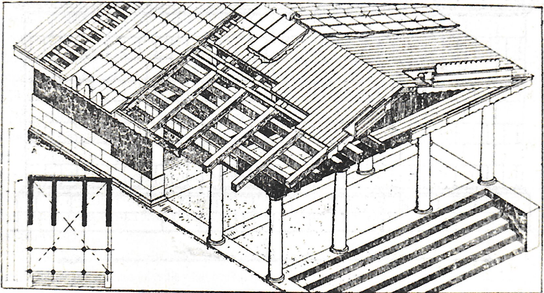
Etruskilaisen temppelin rakenteet. Keksintöjen kirja, WSOY 1938.
