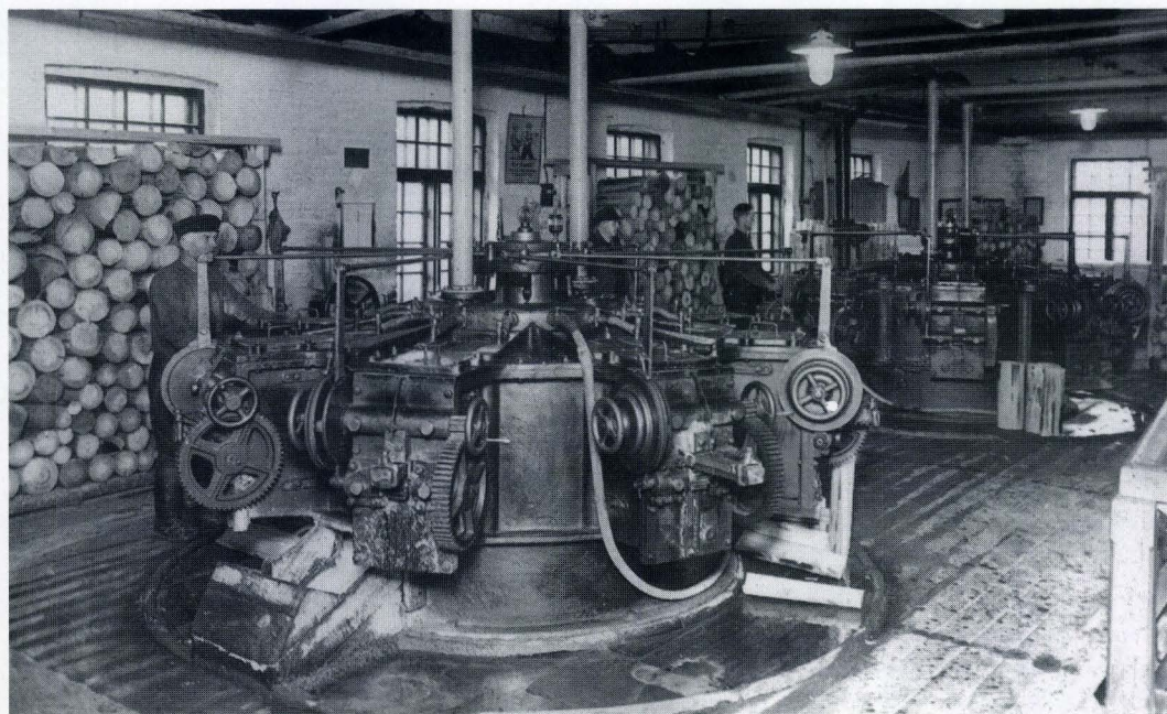
Hiomon pystyakseliset nykäyssyöttöiset kylmähiomokoneet toimitti Karhulan Konepaja 1903. Kuva: Verla.
