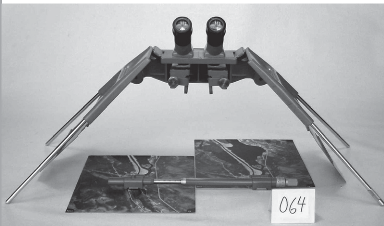
Peilistereoskooppi, jota käytettiin ilmakuvien tarkasteluun aina 1980-luvun lopulle. Kuva: Mobilia, Tiehallinnon esinekokoelma.
