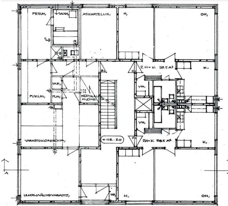
As. Oy Sotkankulman asuinkerrostalon pohjapiirros, maantasokerros. Tässä kerroksessa on kahden kaksion lisäksi taloyhtiön yhteisiä tiloja. Kaksiot käsittävät funktionalistisen asuntoajattelun mukaisesti makuuhuoneen, keittiön, olohuoneen ja pesutilat. Maantasokerroksen yläpuolen kerrosten asunnoissa on parveke. Kuva: Rakennuslupapiirustus, RAVA.
